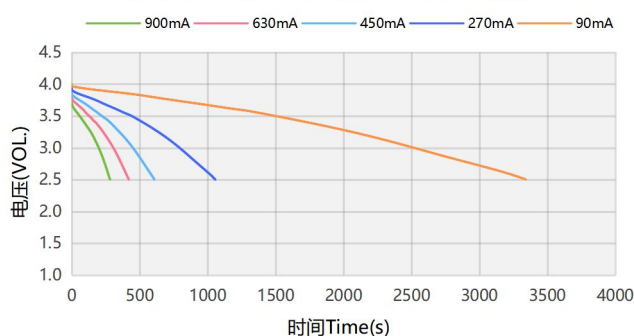
LIB1030Q4R0207 @85°C Dis. Char.
