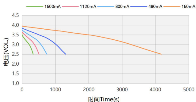
LIB1620Q4R0407 @85°C Dis. Char.
