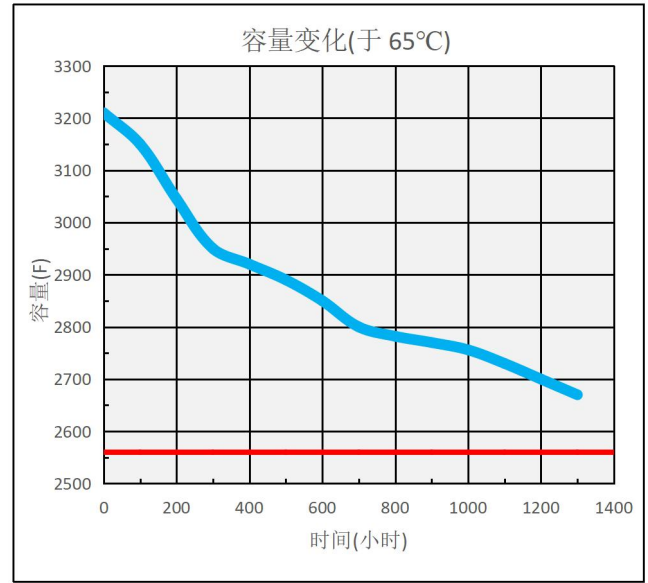
图 1: 加速老化容量性能
