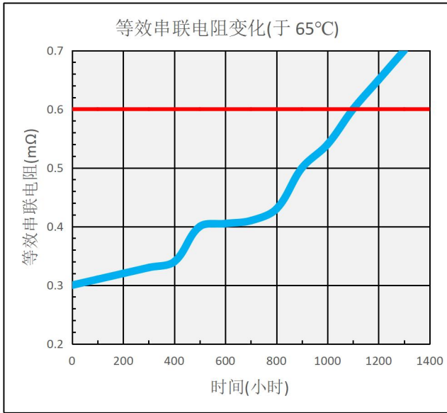
图 1: 加速老化 ESR 性能
