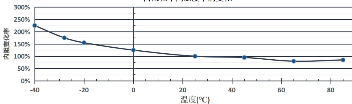
内阻在不同温度下的变化
